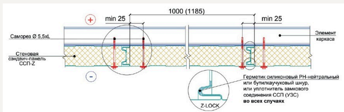
Узел замка стеновых панелей Z-Lock
