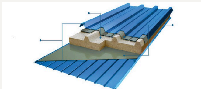
Оцинкованная сталь с полимерным покрытием, утеплитель, клей
