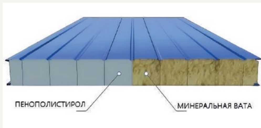
Панели с пенополистиролом и минеральной ватой
