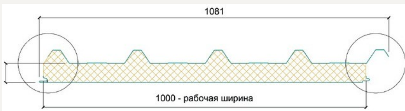
Сечение кровельной панели. 1000 мм — рабочая ширина
